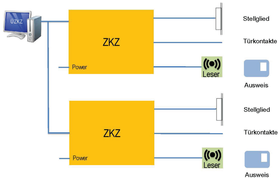
Grafik: Anlagen mit Entscheidungsintelligenz am Zutrittspunkt und zentraler Bedienung
