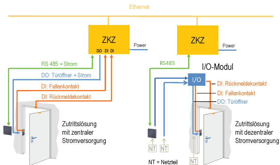
Grafik: Gegenüberstellung von Zutrittslösungen mit zentraler oder dezentraler Stromversorgung
