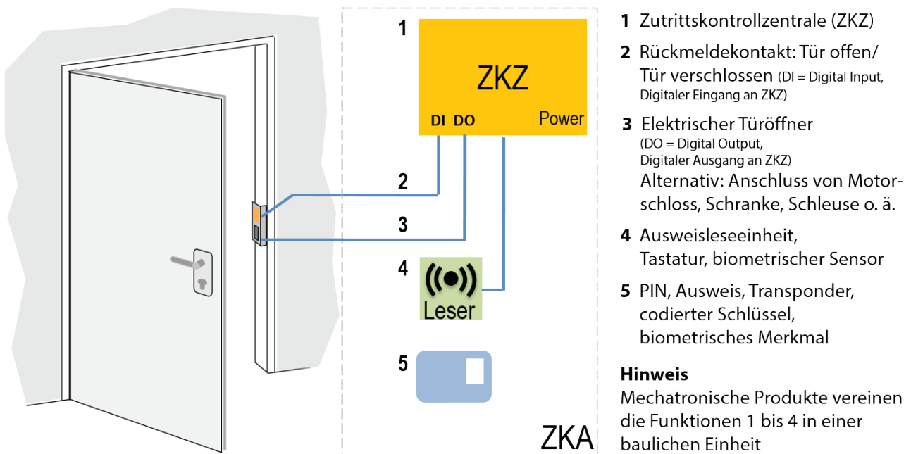
Abb. 1: Grundtyp einer Zutrittskontrollanlage
